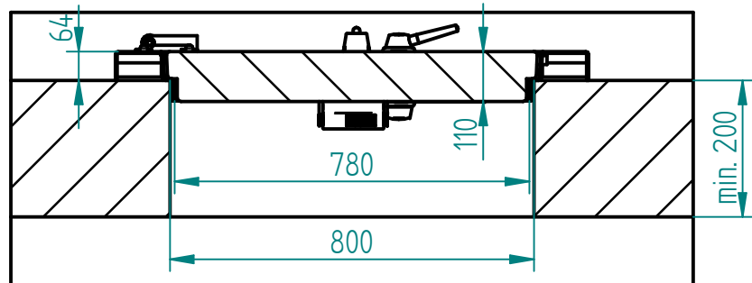
Schnitt B-B
