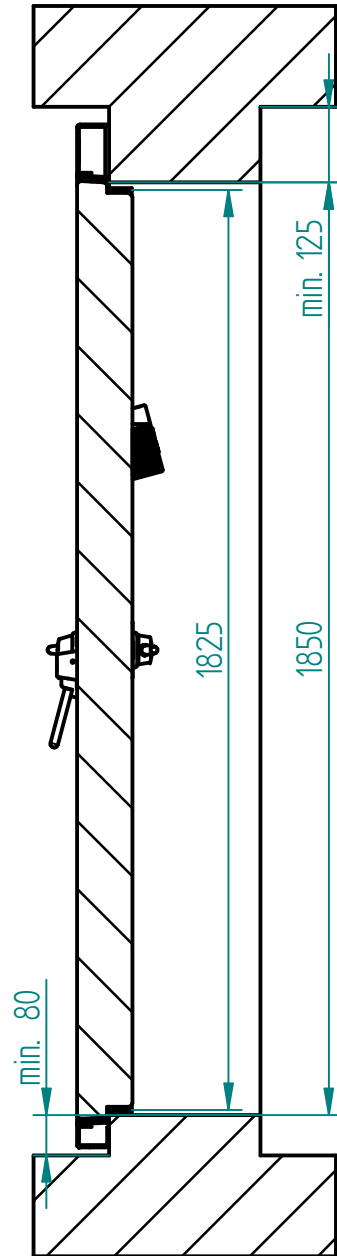
Schnitt A-A
